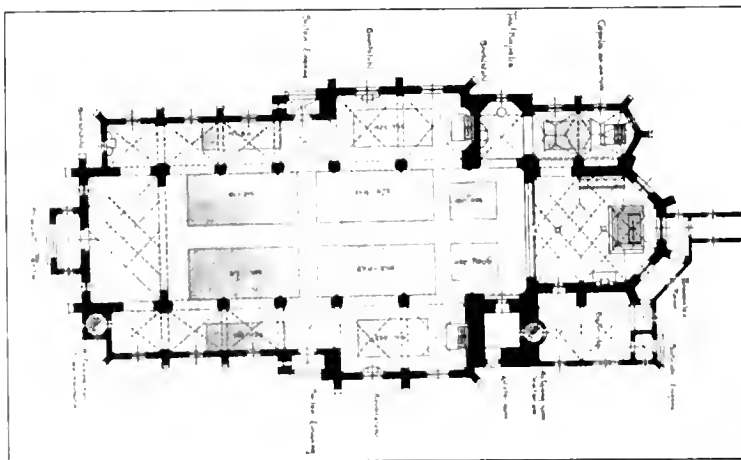
MOTTO -QUERSCHNITT GRUNDRISSE Nr. 15, Text S. 11, vgl. Nr. 12 und 20
